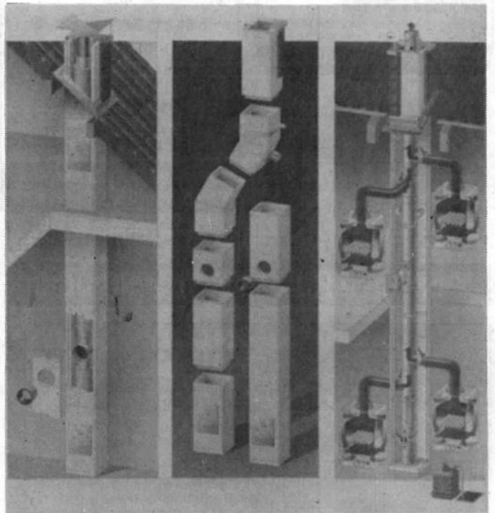
Raab-Trockenbausysteme für den Schornsteinbau. Von links nach rechts: Universalschornstein, System-Abgasleitung, LA-System. Foto: Joseph Raab GmbH & Cie KG
