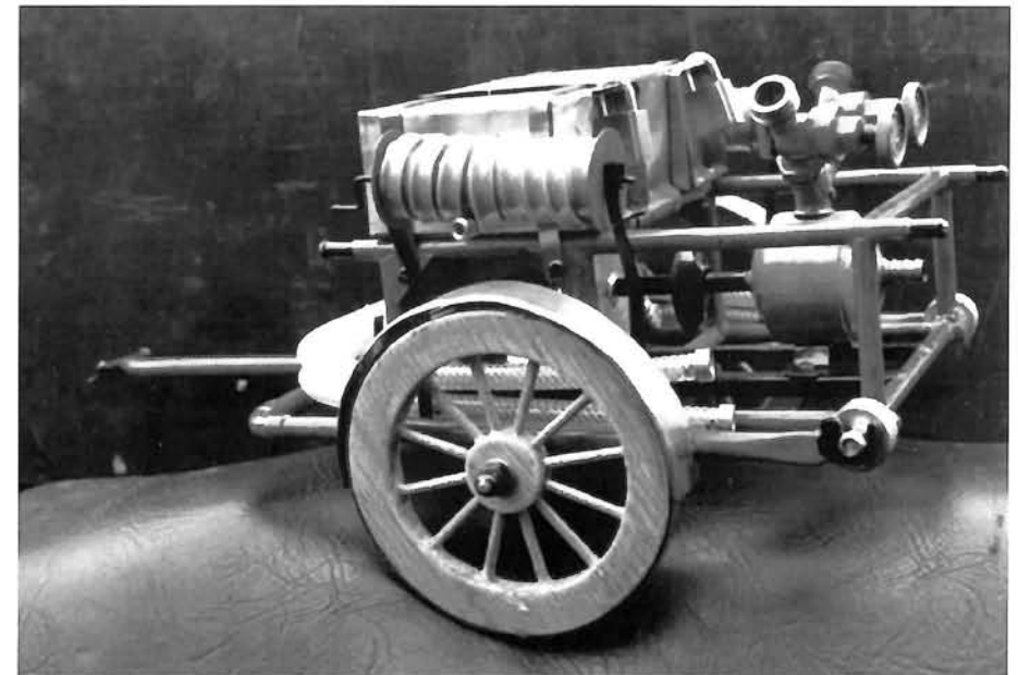
Modell der 1. Motorspritze aus 1928, gebaut von Adolf Seitz
